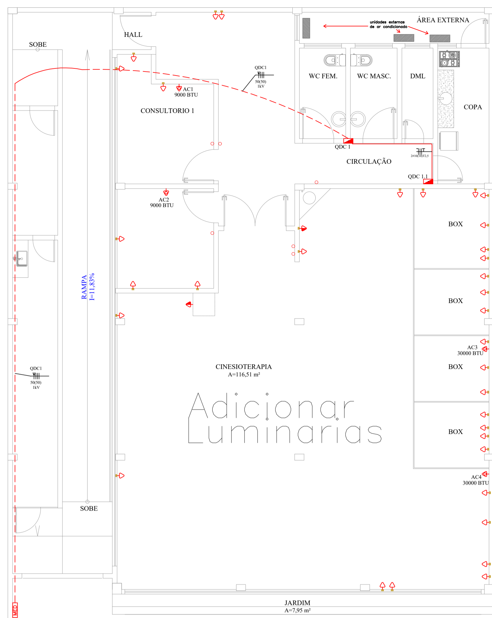
1 PLANTA BAIXA 1º PAV. (Térreo) - Existente ESCALA : 1/75
