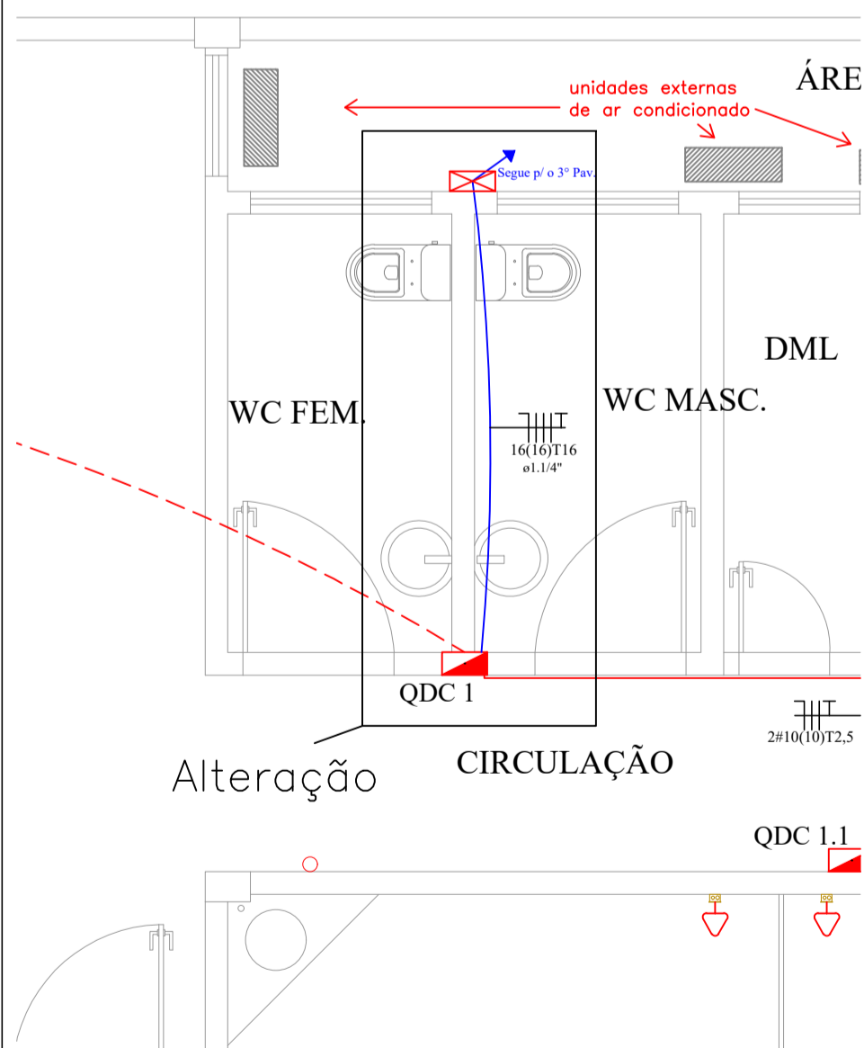
2 ALTERAÇÃO NO 1º PAV. (Térreo) SEM ESCALA
